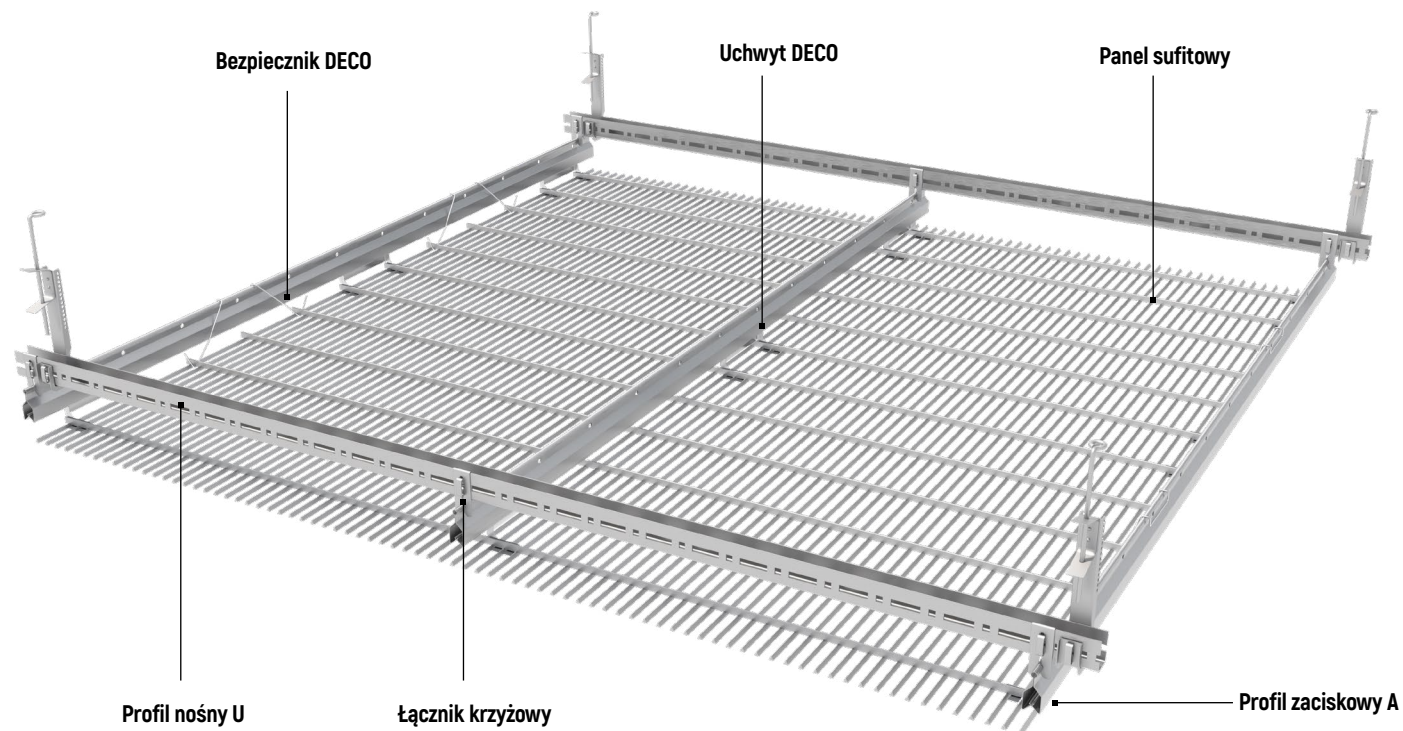
układ krzyżowy dwupoziomowy
