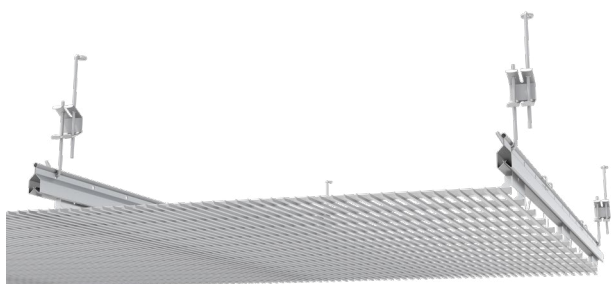
układ równoległy jednopoziomowy
